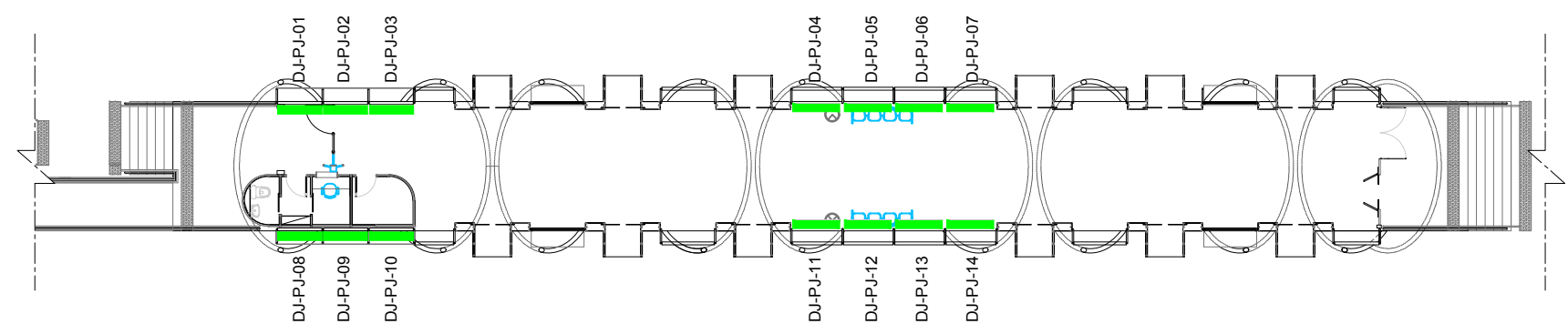
01 PLANTA BAIXA / PLATAFORMA ESC.: 1/15
